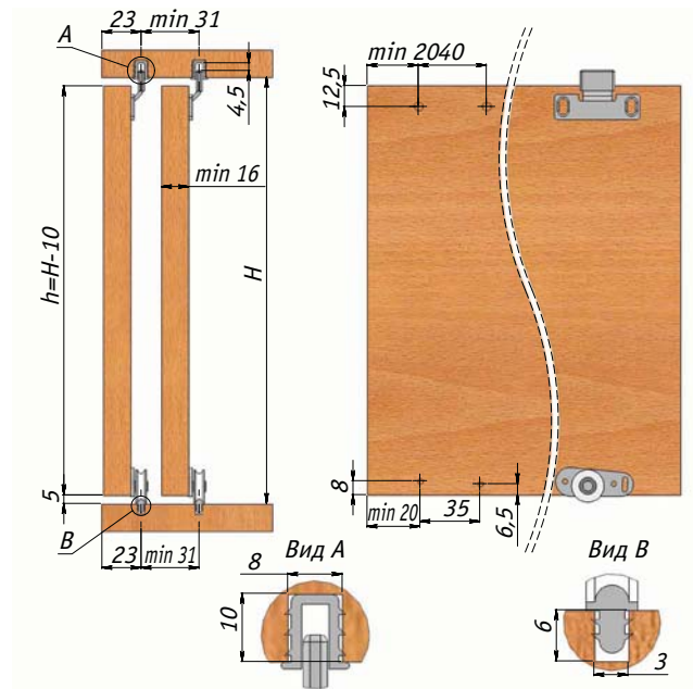
Схема для расчетов и сборки дверей из ДСП с врезными направляющими
