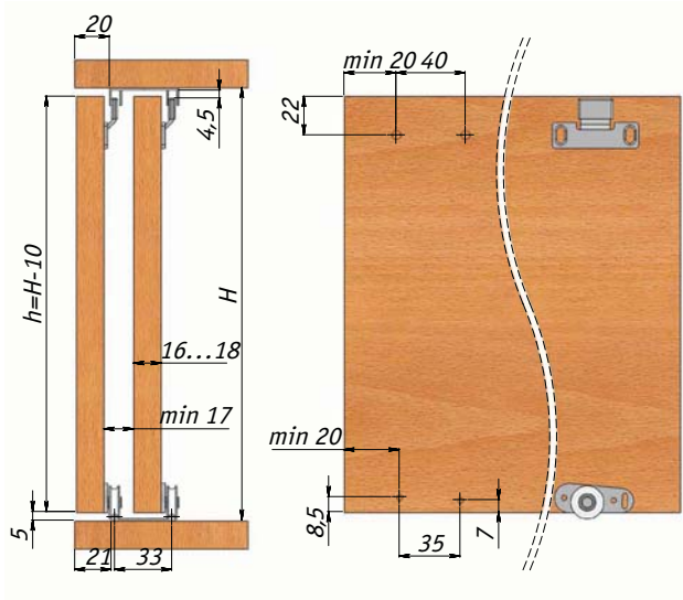
Схема для расчетов и сборки дверей из ДСП с двойными направляющими
