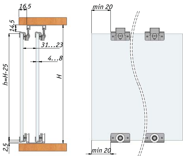
Схема для расчетов и сборки дверей из стекла с накладными направляющими
