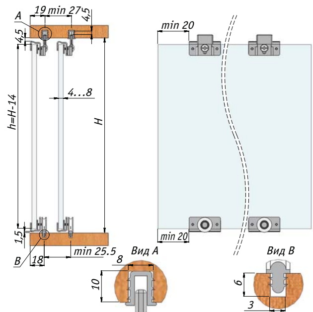
Схема для расчетов и сборки дверей из стекла с врезными направляющими
